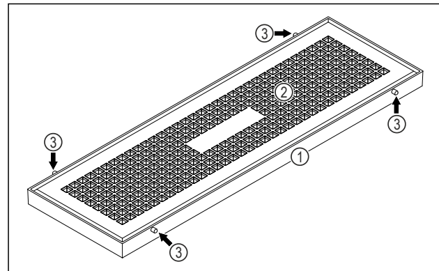
Fig. 108 Ілюстративне зображення, водяна камера (1) Чаша для води (3) Пробка (2) Кришка
