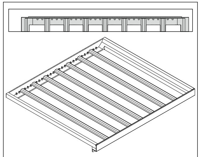
Fig. 103 Розташування планок для максимальної кількості пляшок.
